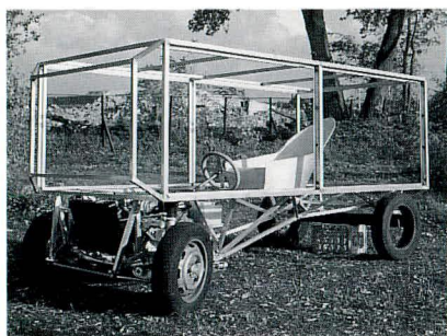
DE VIERKANTE AUTO 1994 Variomatic sport 1100 cc, aluminium. Gereed, november 1994. Ruim en open - Eenvoudig - Goedkoop. THE SQUARE CAR 1994 Variomatic sport 1100 cc, aluminium. Ready, November 1994. Roomy and open - Simple - Cheap.
