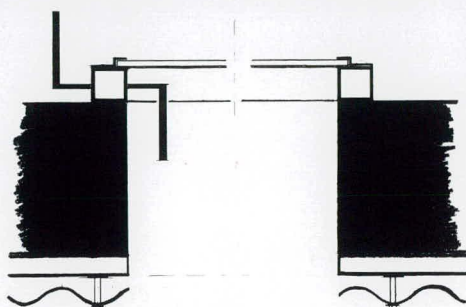
WOONHUIS MET PRAKTIJKRUIMTE, Herdersem België 1984-1988 Bekleed met doorzichtige golfplaten. HOUSE WITH SURGERY, Herdersem Belgium 1984-1988 Covered with transparent corrugated plastic.
